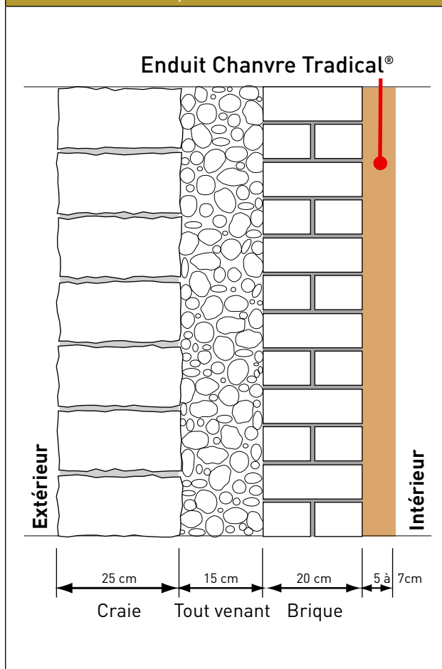
Maison Diocésaine : Coupe verticale d'un mur
